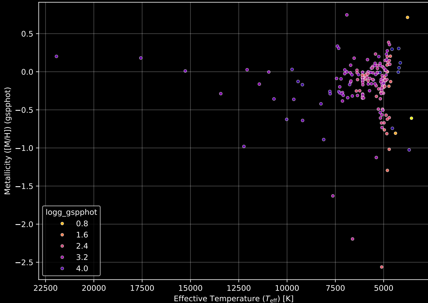
APOGEE DR17 Field: [154+04] Stellar Population Parameters (n= 190)
